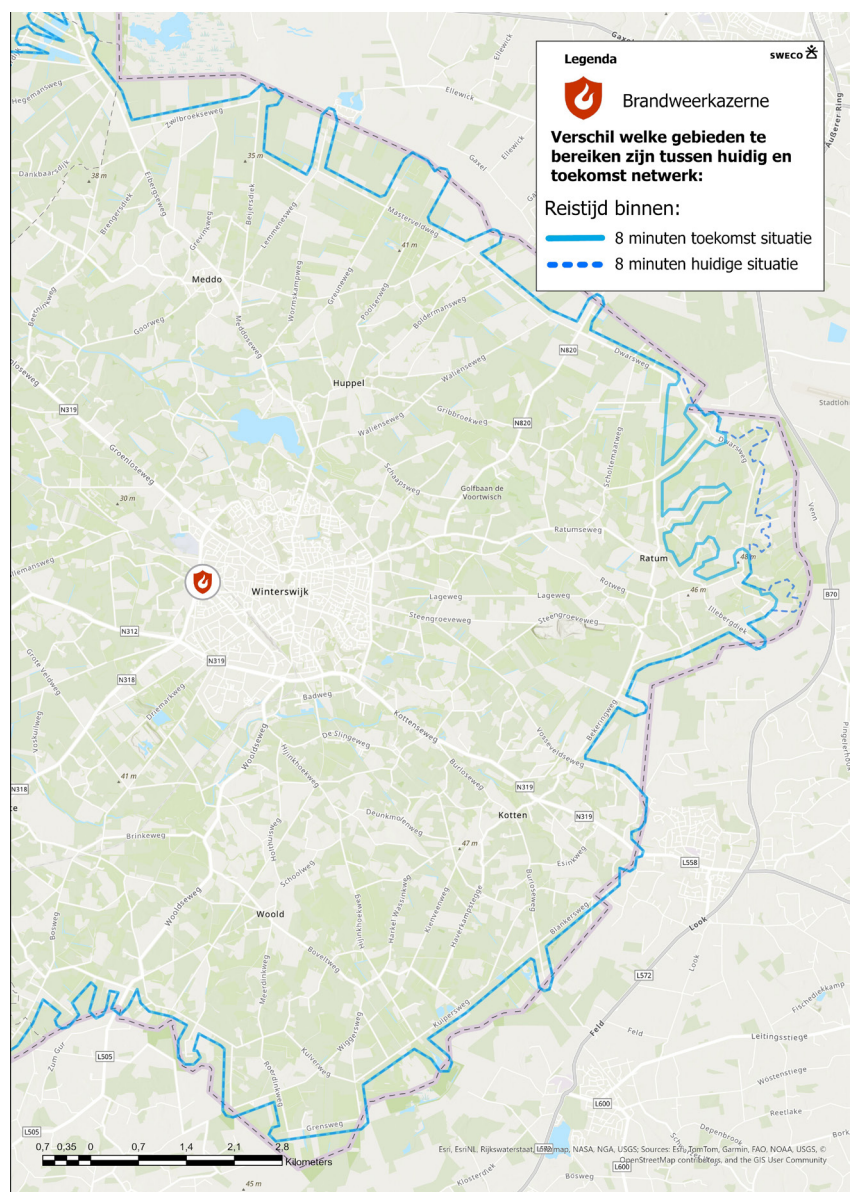
Figuur 7.2: verschil in aanrijtijden vanuit brandweerkazerne Winterswijk met gewijzigde snelheden op hoofdwegen
