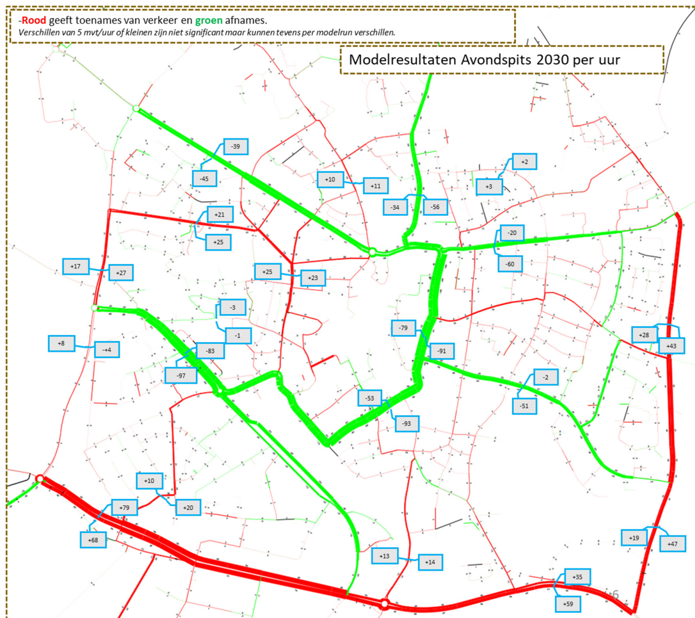
Figuur 7.1: het effect van verlaging maximum snelheid naar 30 km/uur
